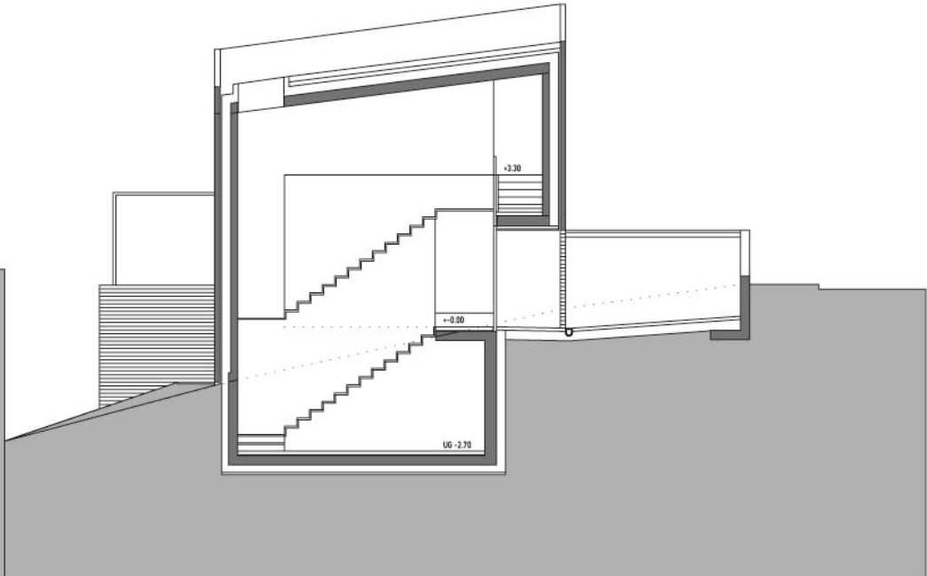
QUERSCHNITT 4
